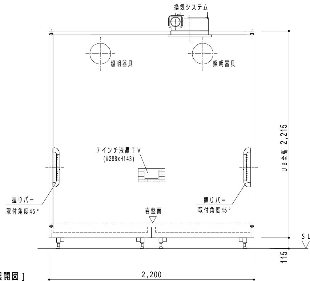
[ C面展開図 ]
