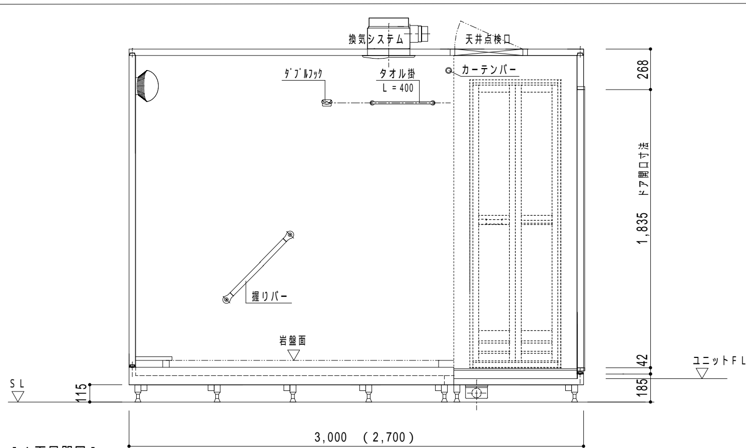
[ A面展開図 ]
