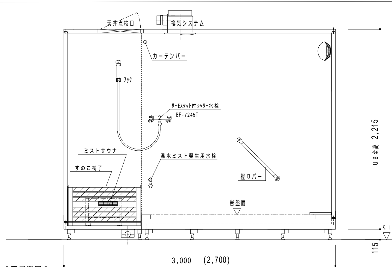
[ C面展開図 ]
